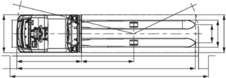
Vista superior OPX-L 16
