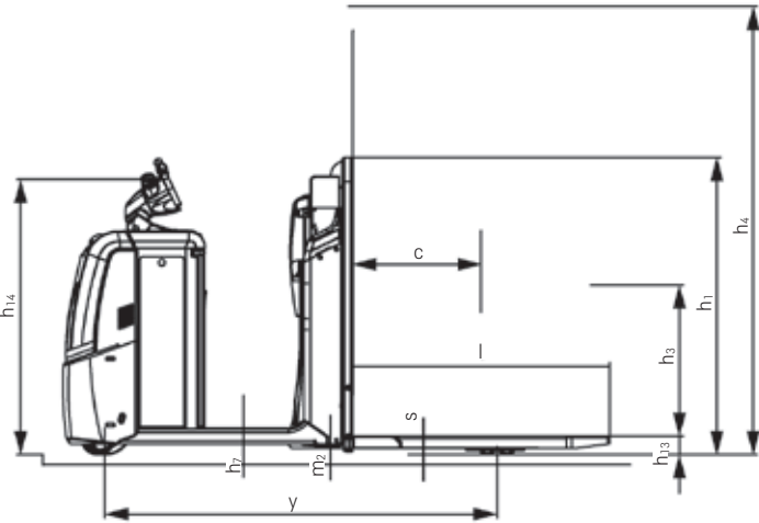
Vista lateral OPX-L 12
