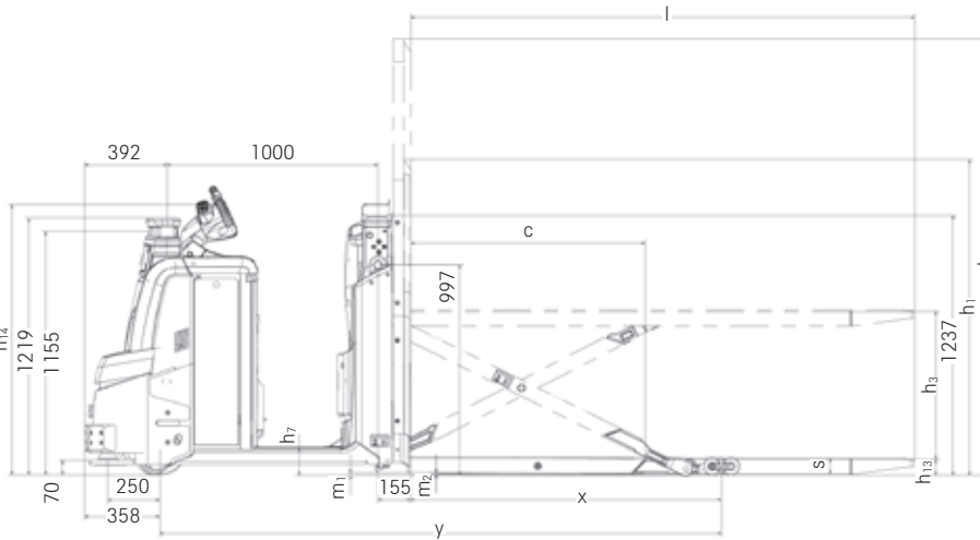
Vista lateral OPX-L 20 S iGo neo
